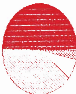
Macrofaune - Bayerel
